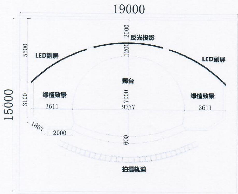
演播厅平面布置图
