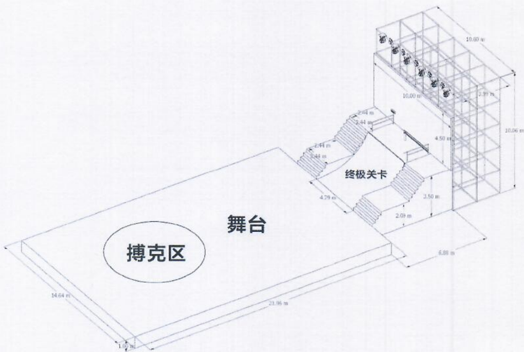
俯视图
