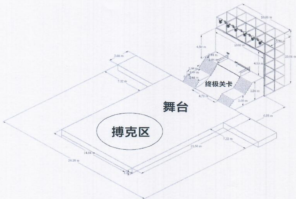
俯视图
