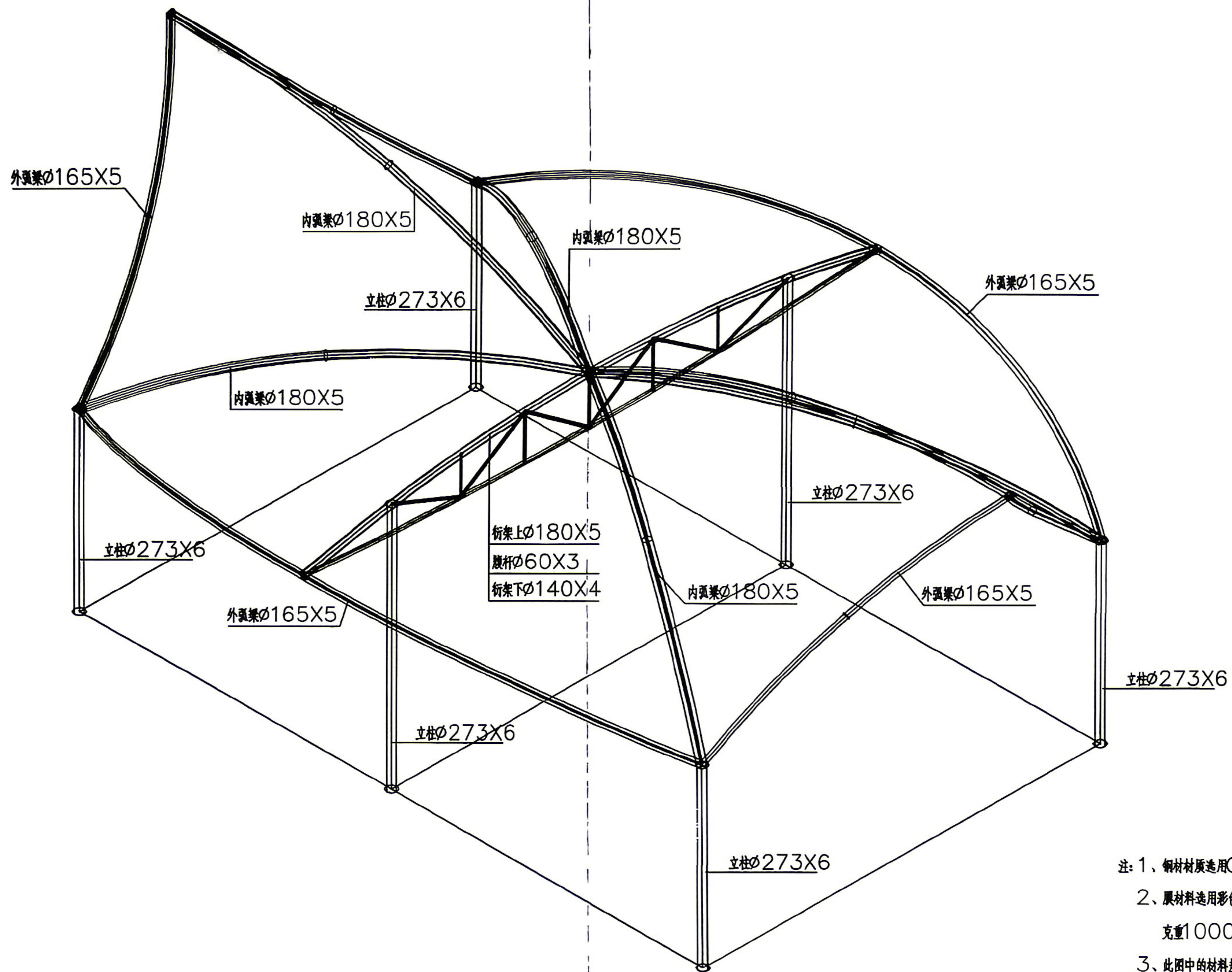
结构规格图
