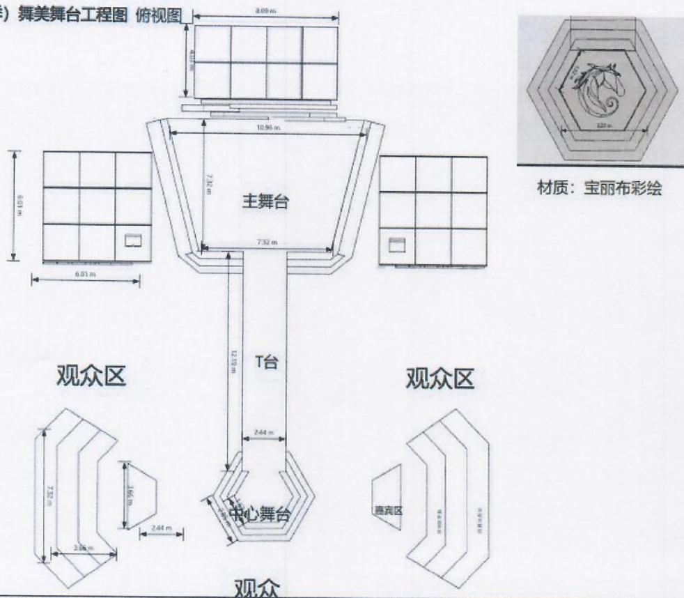
《歌从草原来》（民歌季）舞美舞台工程图 俯视图
